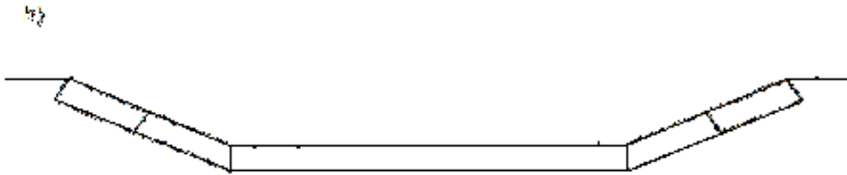
Rys. 7. Materac dostarczony na budowę w formie złożonej skrzynki, którą rozkłada się i usztywnia przegrodami co np. 1,0 m. Wieko dostarczane jest osobno.
